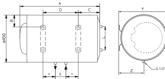
Горизонтальні моделі
